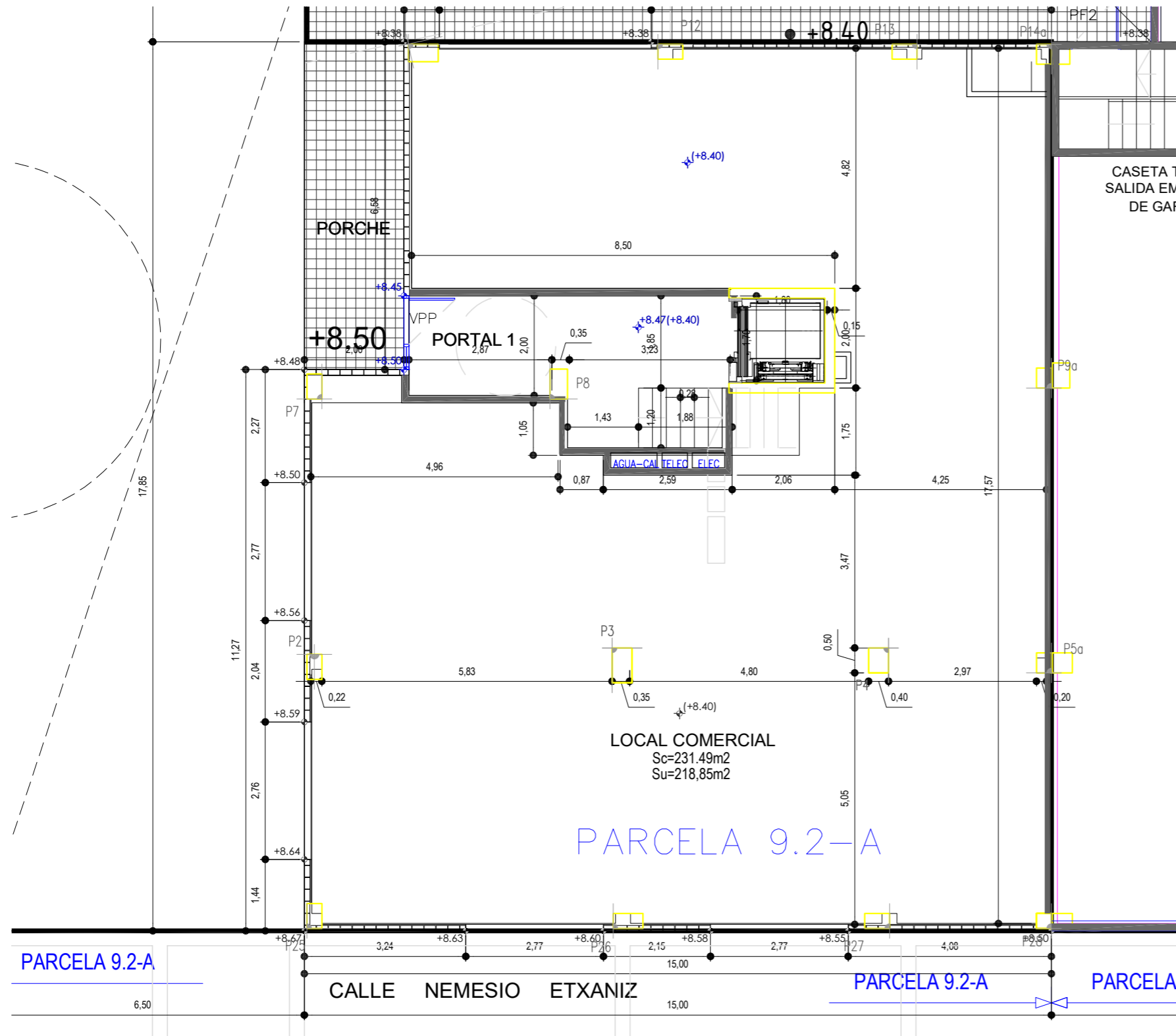
PLANTA DE LOCAL E 1/100 LOKALAREN OINPLANOA
